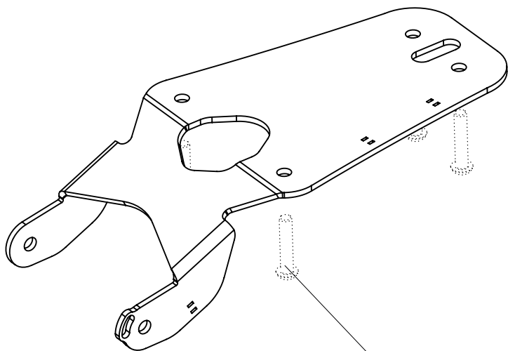
VITE ORIGINALE Original screw
